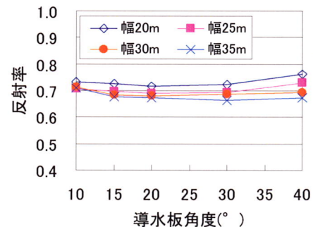
図-9 導水板角度と反射率の関係 (周期30s)
