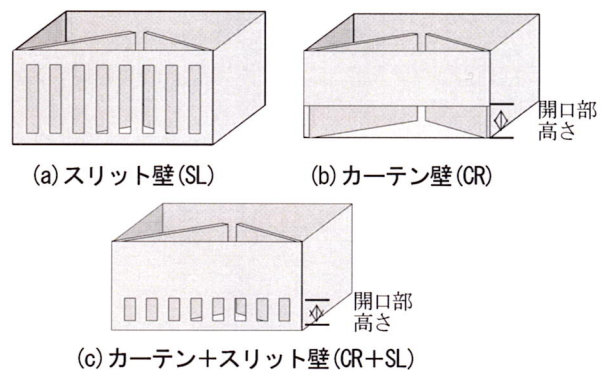
図-15 前面壁形状
