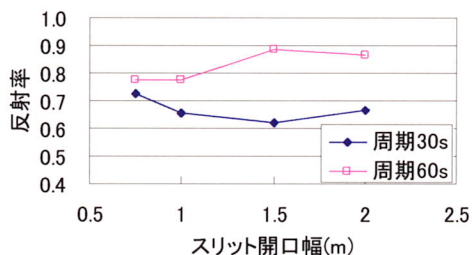
図-12 スリット開口幅と反射率の関係
