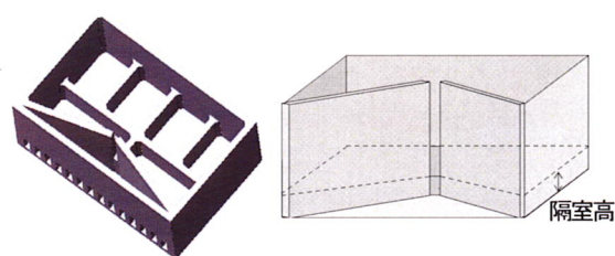
①中詰め用の隔室がある場合(重力式)
