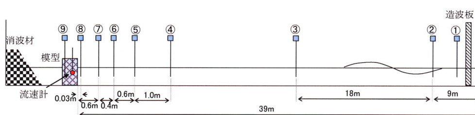
図-2 水理模型実験概略図
