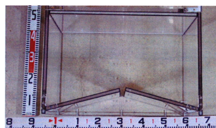
図-4 基本模型(幅20m, 角度15度, 開口幅0.75m)
