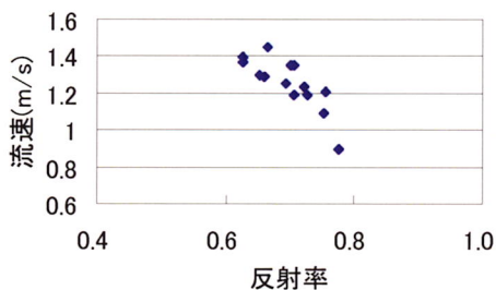
図-13 スリット開口部付近の流速と反射率の関係
