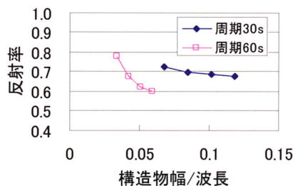
図-8 構造物幅(無次元量)と反射率の関係 (導水板角度15°)
