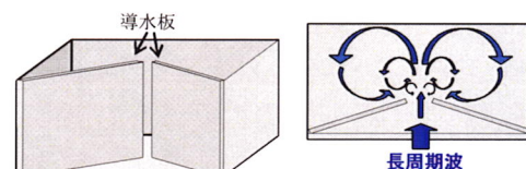
図-1 渦消波タイプの長周期波対策構造物
