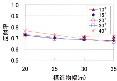
図-6 構造物幅と反射率の関係 (周期30s)
