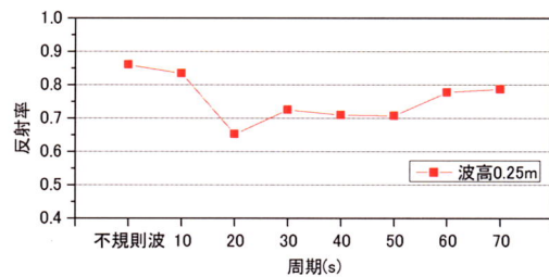
図-14 詳細実験結果
