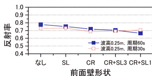
図-16 前面壁形状と反射率
