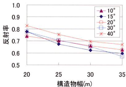
図-7 構造物幅と反射率の関係 (周期60s)
