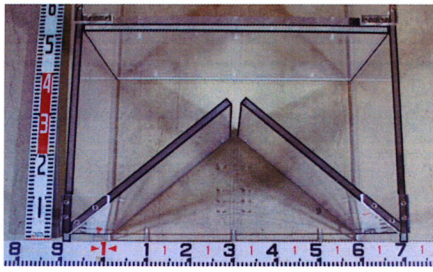
図-5 基本模型(幅20m, 角度40度, 開口幅0.75m)
