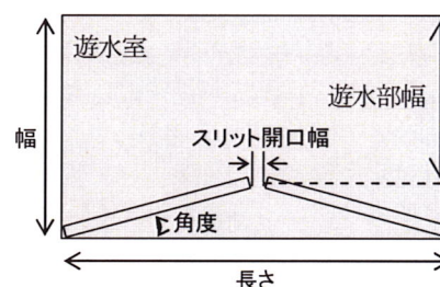
図-3 基本形の模型平面図
