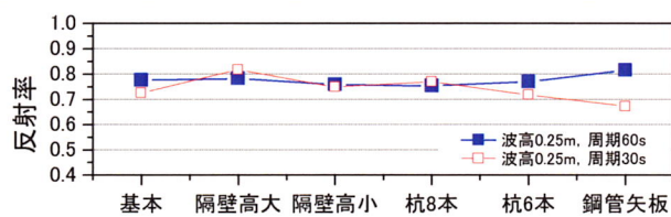
図-18 構造形式別の長周期波低減性能
