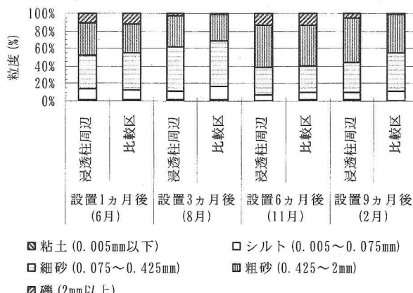
図-9 浸透柱設置後の粒度分布の変動
