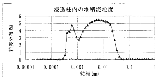
図-12 浸透柱内の堆積泥粒度 (平成16年12月25日～1月25日)
