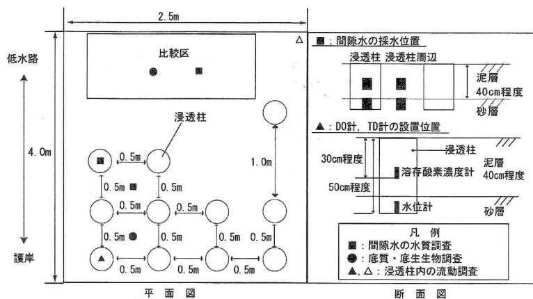
図-5 実験の概要 (浸透柱の設置要領と調査位置)
