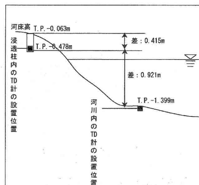
図-6 水位計 (TD計) の設置状況
