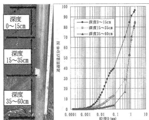
図-3 底質状況および粒度分布
