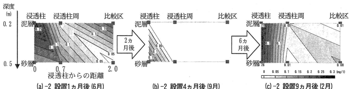
図-10 間隙水内栄養塩の分布変化
