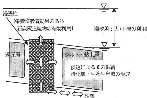
図-1 有機泥の対策方法
