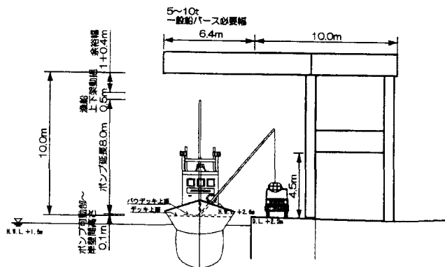
図-7 ほたて桁引き網漁業屋根所要天端高算出の考え方
