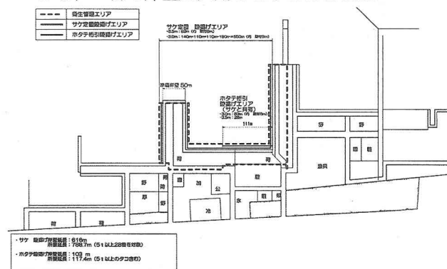
図-3 標準漁港ゾーニング図
