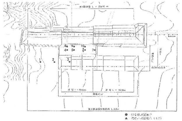
図-2 流速計と付着板の設置位置図
