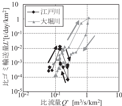
図-5 比流量と比ゴミ輸送量の相関図
