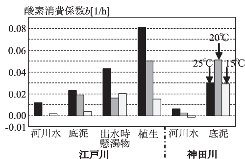
図-7 各有機物サンプルの酸素消費係数 b
