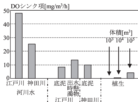
図-8 DOシンク項(式(1)第1, 2, 3項)
