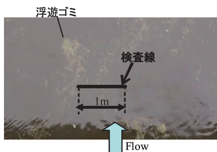
図-2 実際の撮影画像と解析方法の概要
