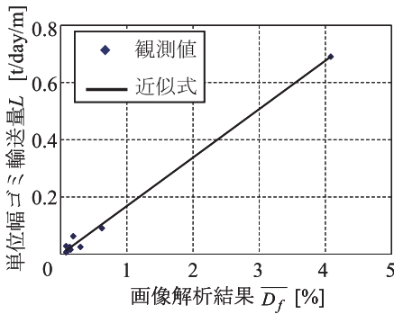
図-4 単位幅ゴミ輸送量の観測値と画像解析結果の比較
