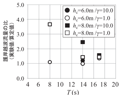
図-8 実験値と算定値による護岸越波流量の比較
