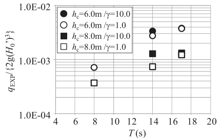
図-5 「直立護岸」に対する平均越波流量
