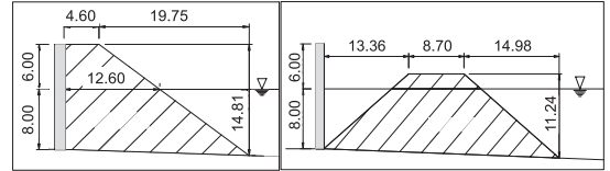
(a)「消波護岸」 (b)「透過離岸堤を有する直立護岸」
