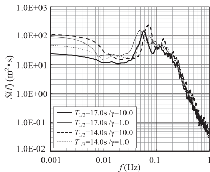
図-6 直立護岸前面におけるスペクトル密度
