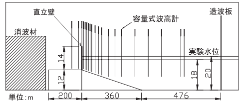
図-3 実験水槽(断面図)
