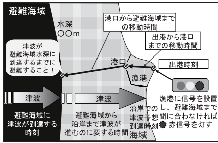
図-4 陸上滞在時の漁船避難の考え方
