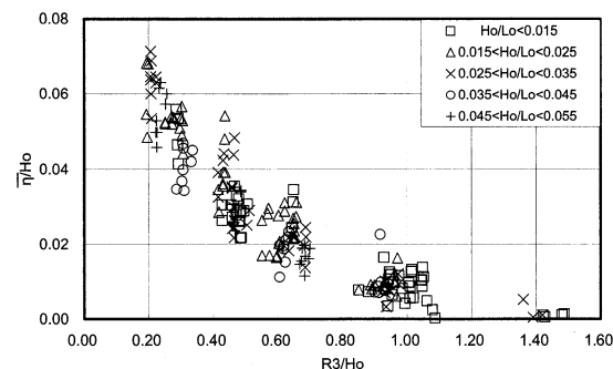
図-4 トラップ式ダブルリーフによる水位上昇量特性
