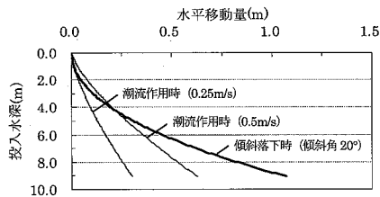
図-11 水平移動量解析結果
