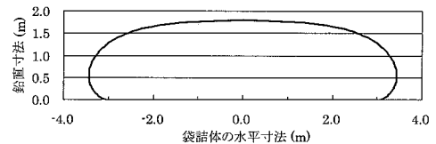
図-9 袋詰体予測形状
