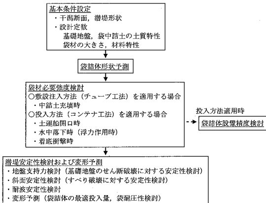
図-3 袋詰体を用いた潜堤の設計手法の提案
