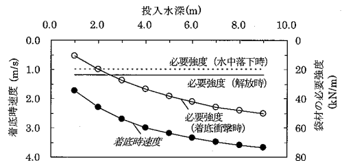
図-10 着底時速度および袋材必要強度解析結果
