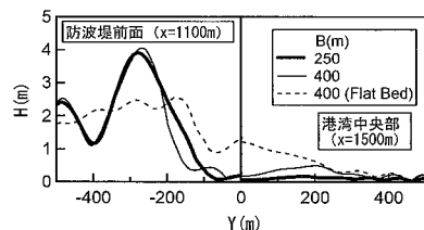
図-12 防波堤開口径による波高分布の変化
