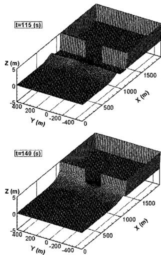
図-13 孤立波に対する数値解析結果(水面変位の空間分布)
