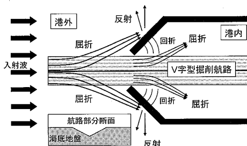
図-1 V 字型航路掘削による波浪制御の概念図
