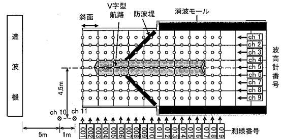
図-5 港内波高分布の計測位置
