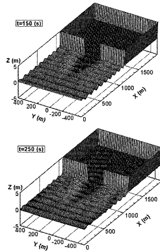
図-11 規則波に対する数値解析結果 (水面変位の空間分布)
