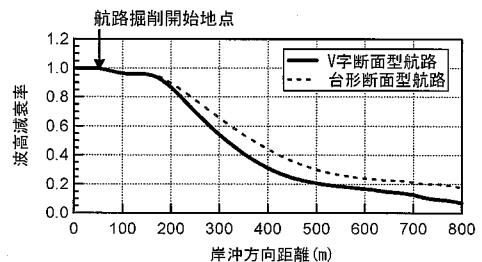
(b) 航路中央部における波高の岸沖方向変化
