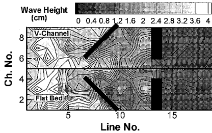
図-8 二重防波堤配置の場合の波高分布
