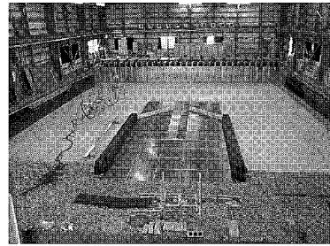
図-4 実験装置および港湾模型の概要
