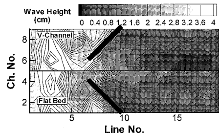
図-6 港内波高分布の計測値
