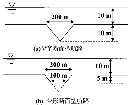
図-2 航路断面 (沿岸方向) の設定
