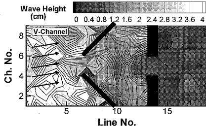
図-9 斜め入射の場合の波高分布 (入射角 10 度)
