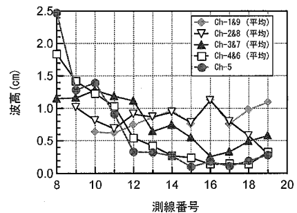
図-6 港内波高分布の計測値
