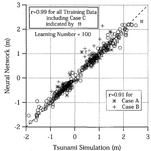
図-8 訓練回数を制限したときの全5地点におけるニューラルネットワークによる予測値と津波シミュレーション値の比較
