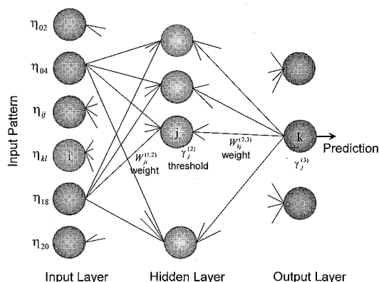
図-1 階層型ネットワーク
