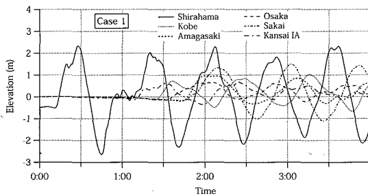
図-3 規模を考慮した Ando モデルによる津波計算結果
