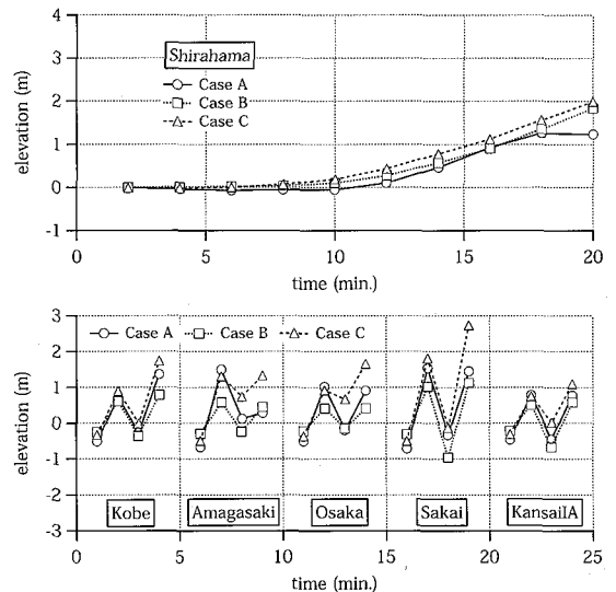
図-5 テストケースの時間波形と水位低下量, 上昇量
