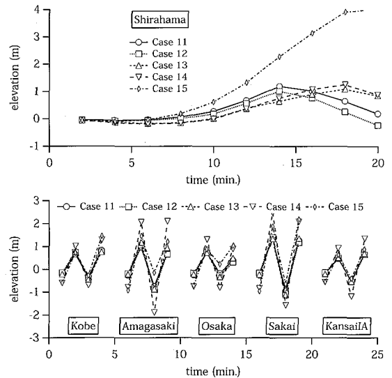
図-4 白浜観測塔における時間波形と大阪湾内5地点における水位低下量と上昇量
