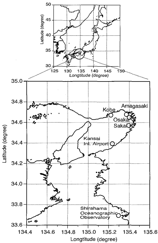
図-2 白浜観測塔と津波予測対象地点
