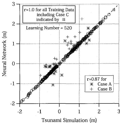
図-7 訓練回数を自動化したときの全5地点におけるニューラルネットワークによる予測値と津波シミュレーション値の比較
