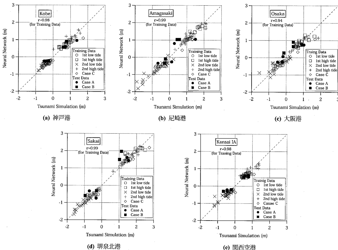
図-6 ニューラルネットワークによる予測結果
