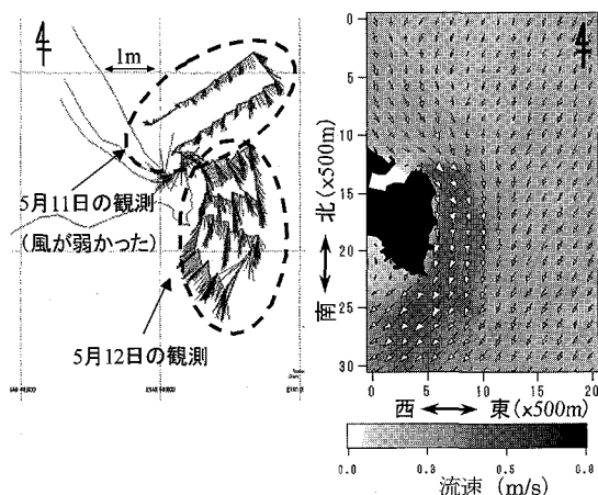
図-9 流速図 (左: 観測値, 右: 計算値)
