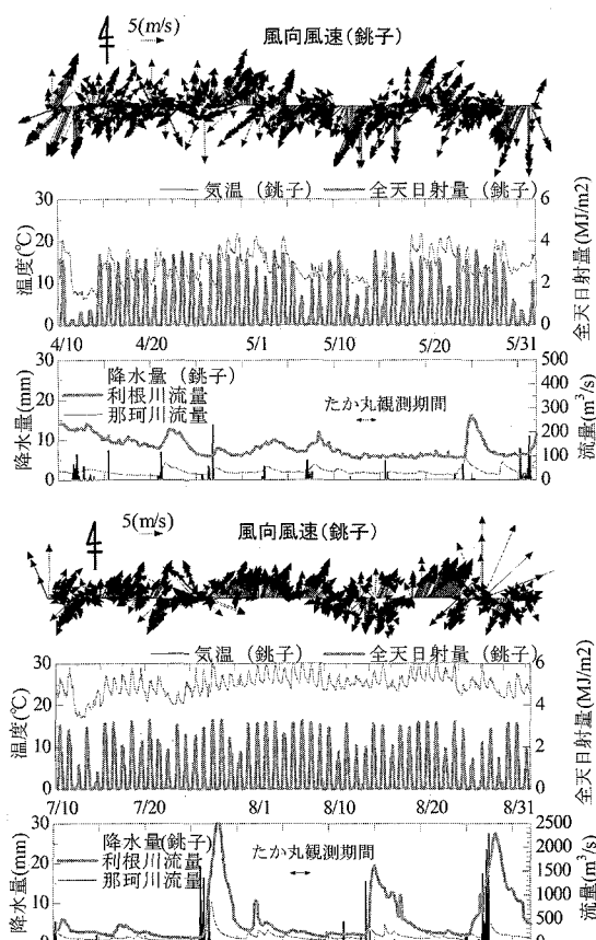
図-8 気象及び流量の時系列 (上: 春季, 下: 夏季)
