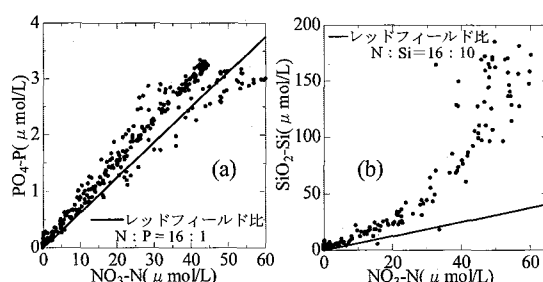
図-4 栄養塩濃度の相関図(JODC データより)
