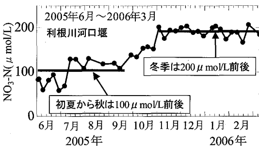
図-6 利根川の硝酸塩濃度の時系列（毎週採水）
