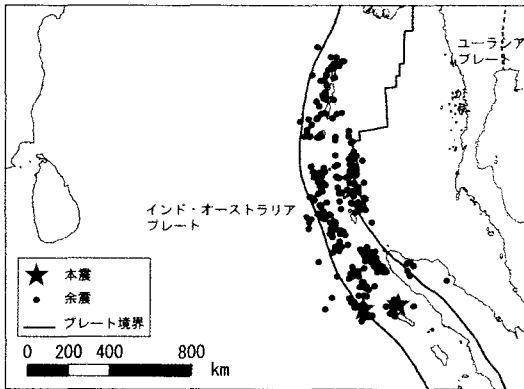
図-2 12月26日の本震の震源と余震分布
