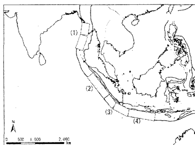
図-9 スンダ海溝沿いの想定地震断層
