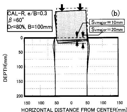
(b) \beta=60^\circ 地盤, CAL-R 試験
