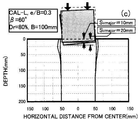
(c) \beta=60^\circ 地盤, CAL-L 試験
