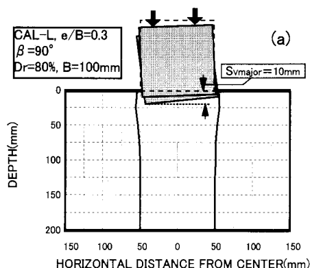
(a) \beta=90^\circ 地盤, CAL-L 試験
