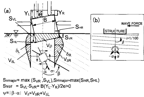
図-3 変形の定義
