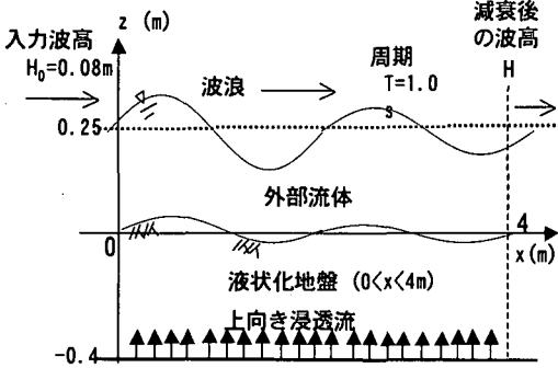
図一4 液状化地盤による波高減衰実験 (高橋ら, 1994) における波浪・地盤条件
