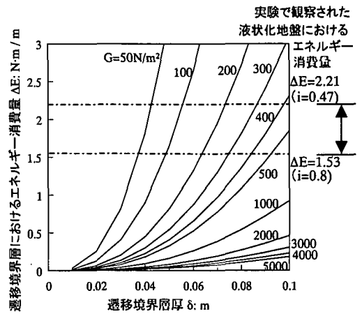
図一5 遷移境界層におけるエネルギー消費量の予測結果と高橋らの実験 (1994) で観察された液状化地盤におけるエネルギー消費量との比較
