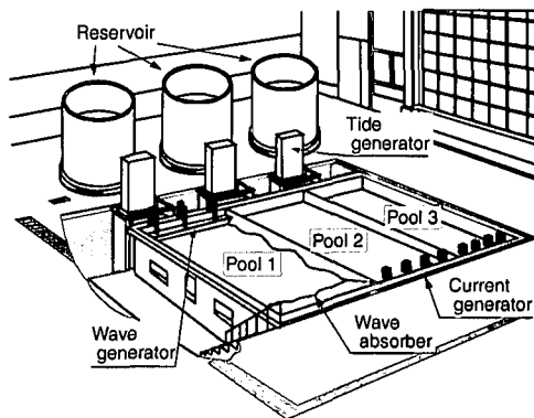
図一 干潟実験施設の見取り図
