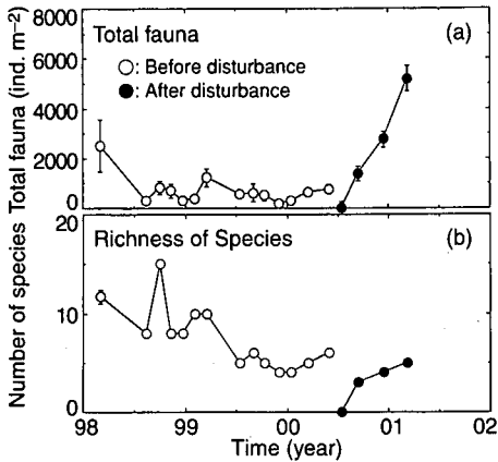
図-5 堆積物の攪拌前(○)および攪拌後(●)における底生動物(マクロベントス)の総個体密度(a)および種類数(b)の経時変化
