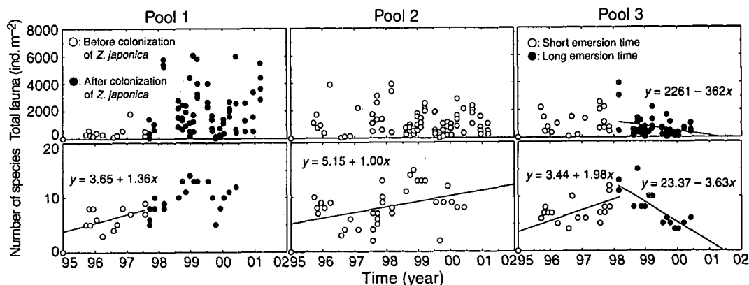
図-3 各実験水槽における底生動物（マクロベントス）の総個体密度（上段）および種類数（下段）の経時変化。近似直線は統計的に有意（ P < 0.05 ）。
