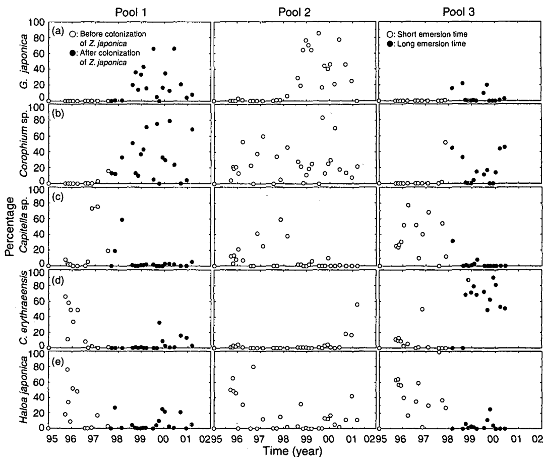
図-4 底生動物（マクロベントス）の優占5種における優占率（%）の経時変化。(a)：ニホンドロソコエビ；(b)：ドロクダムシ；(c)：イトゴカイ；(d)：コケゴカイ；(e)：ブドウガイ。
