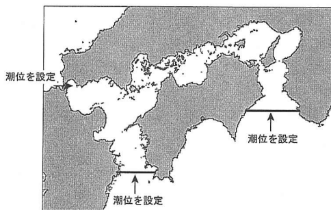
図-5 境界条件の入力地点
