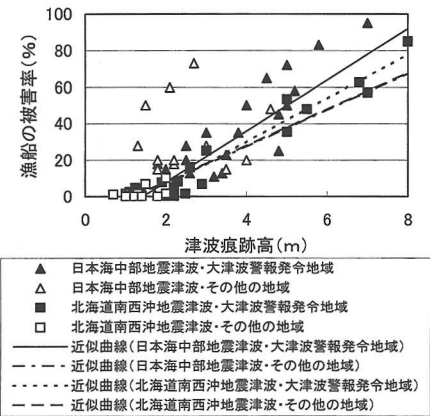
図一1 津波痕跡高と漁船被害率の関係
