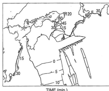
(b) 津波高が1.5 mに達するまでの時間
