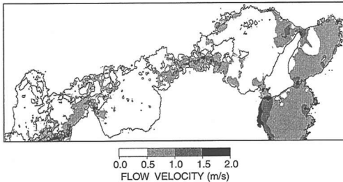
図-9 最大流速分布 (M8.4, 潮汐: Case 2)
