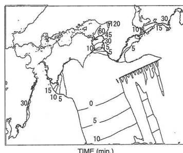
(d) 津波高が1.5 mに達するまでの時間 (断層：東)
