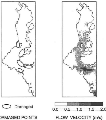
図一3 実際の被害発生箇所 (左) と数値計算で得られた大船渡湾の流速 (右)
