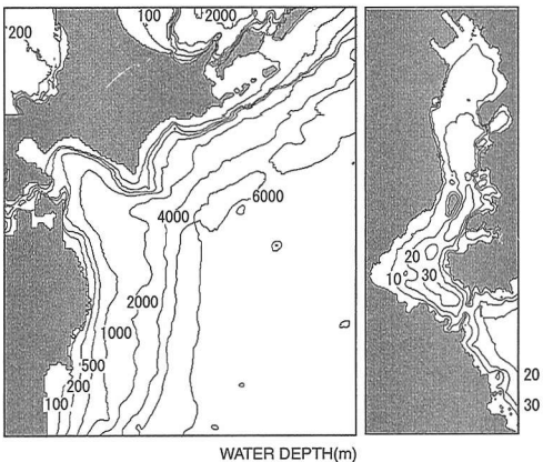
(a) 大領域 (b) 小領域
