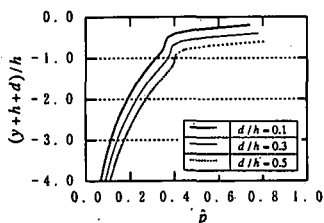
図-4 無次元変動間隙水圧振幅の鉛直方向変化
