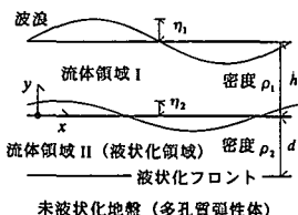
図-1 解析領域
