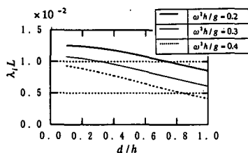
図-3 減衰パラメータ \lambda_i の評価 ( h=10 m の場合)
