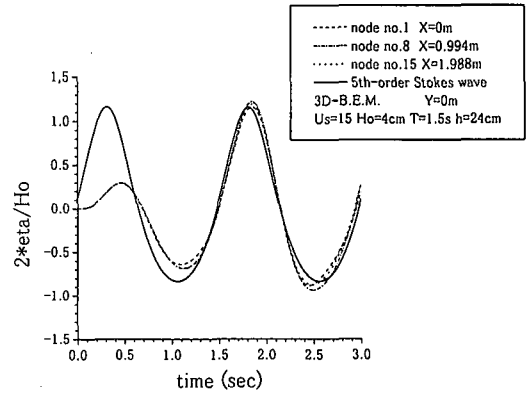
図一3 3D-B.E.M.による水面変動とストークス波の第5次近似解との比較
