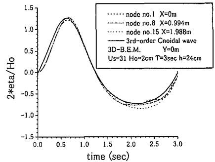
図一4 3D-B.E.M.による水面変動とクノイド波の第3次近似解との比較
