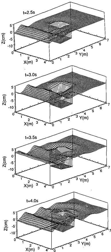
図-6 3D-B.E.M.による自由水面と浮体没水部の3次元空間変動鳥瞰図 ( U_s=15 , H_o=4 cm, T=1.5 s, h=24 cm, K=4 kgf/cm/基)
