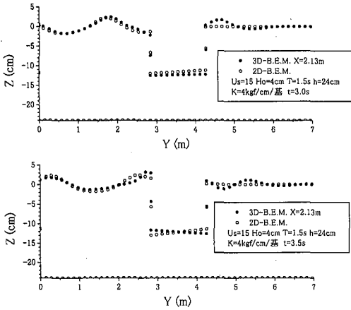
図-5 3D-B.E.M.と2D-B.E.M.との要素節点の空間変動の比較例
