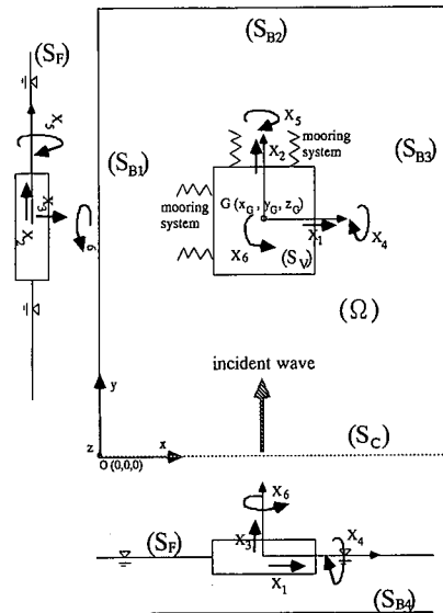
図一 計算領域の座標系と浮体運動の定義
