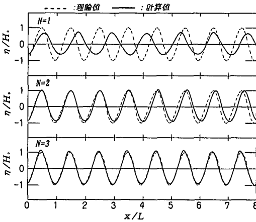
図—6 高波数域 ( kh=6.0 ) における水平床伝播計算
