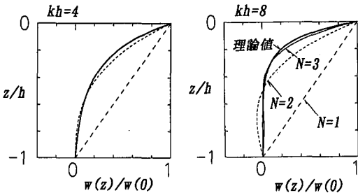
図-3 線形鉛直流速の鉛直分布
