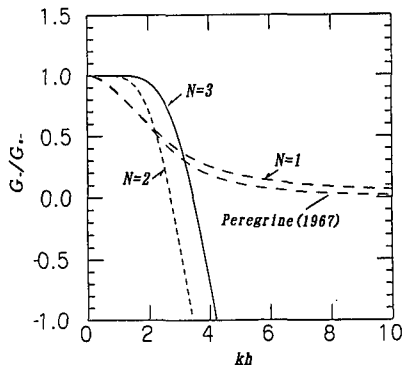
図-5 2次非線形干渉特性 (subharmonics)
