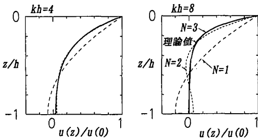
図-2 線形水平流速の鉛直分布
