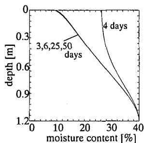
図-10 土壌中の水分 (run-6)
