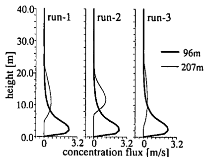
図-9 植生帯前面部 (96 m) と後縁部 (207 m) での無次元塩分濃度フラックス Cu の鉛直分布
