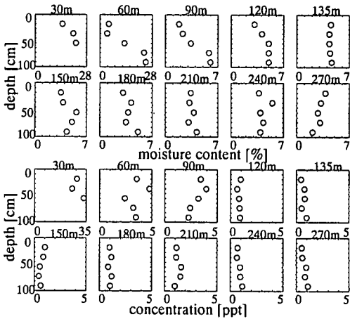
図-3 土壌水分量(上)と土壌塩分濃度(下)の分布
