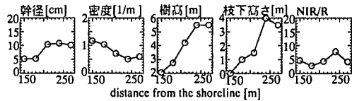
図-2 マツの幹の直径, 密度, 樹高, 枝下高さ, NIR/R
