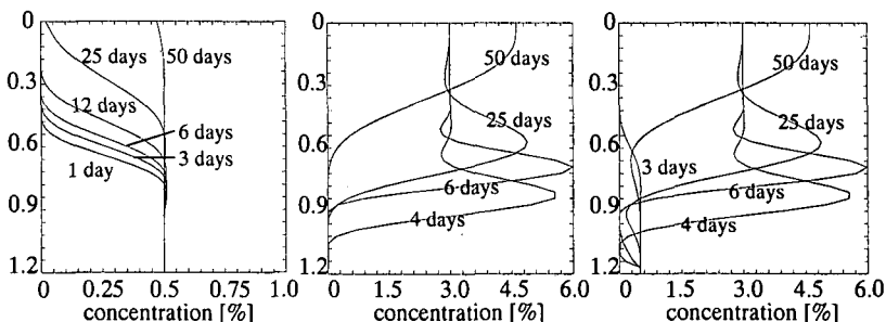
図-11 塩分濃度分布 (左から run-4, run-5, run-6)
