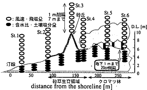
図一 観測機器等の配置・地形断面
