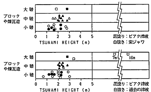
図-6 没水深とブロックや煉瓦造家屋の被害程度の関係
