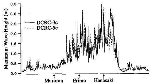
図-4 DCRC-5cおよびDCRC-3cによる計算結果の比較
