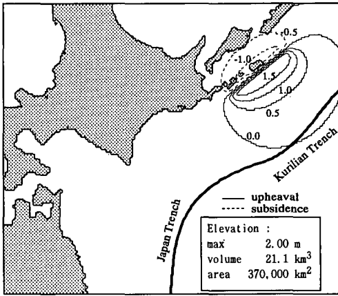
図-1 DCRC-3cによる津波初期波形
