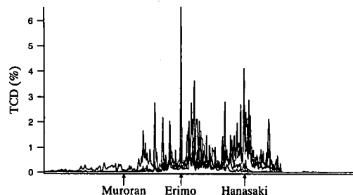
図-7 既往地震津波による TCD 分布の比較
