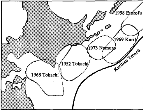
図-5 既往地震による津波初期波形
