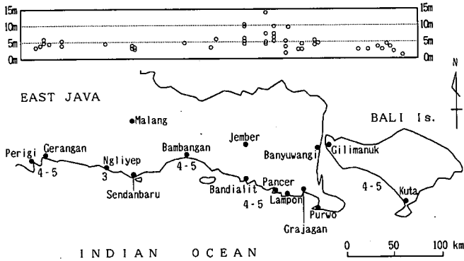
図一2 各地の津波打ち上げ高と震度
