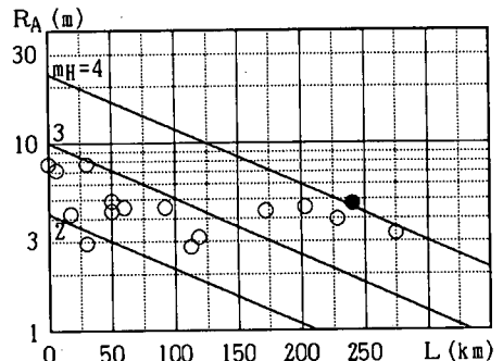
図一3 打ち上げ高と投影点間距離の関係
