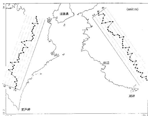
図-5 最大水位の地域分布
