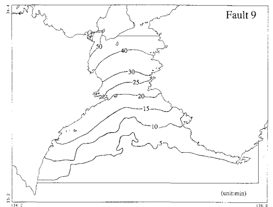
図-3 最短到達時間の等時曲線
