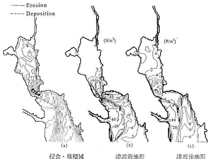
図-7 海底変動図と全計算時間での最大せん断力
