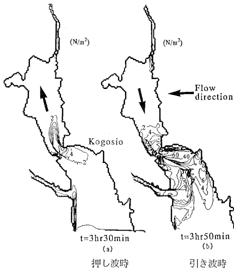
図—8 押し波時と引き波時におけるせん断力
