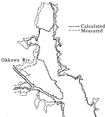
図—9 計算と痕跡から分かる浸水域の比較
