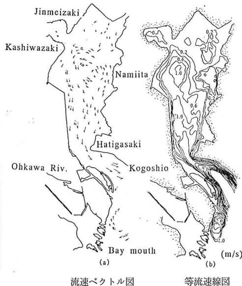
図-1 流速の測定結果
