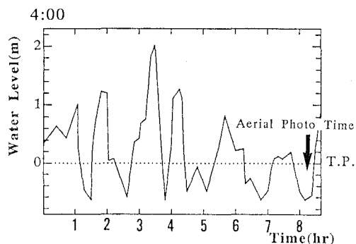
図-3 湾口に与える入力波
