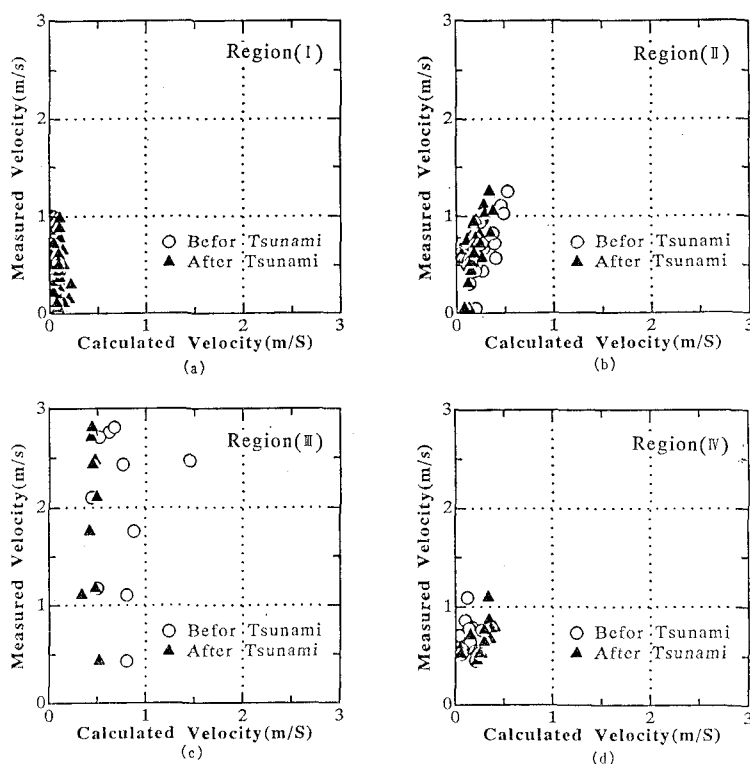
図—5 流速の計算値と測定値の比較
