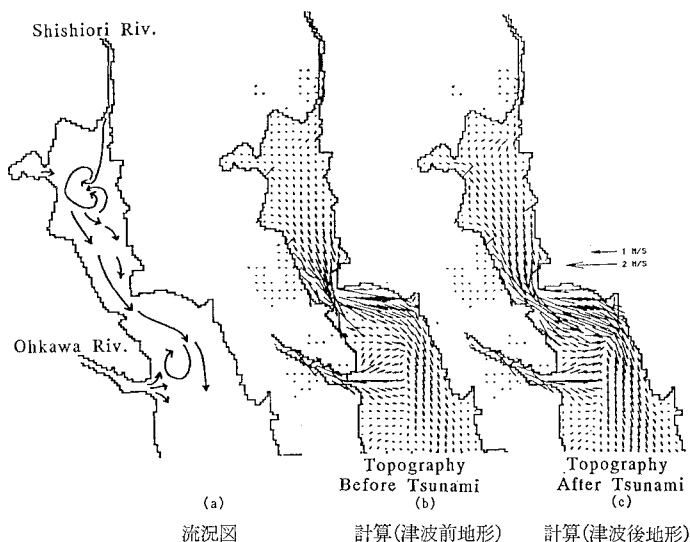
図-4 測定からの流況と計算による流速ベクトル
