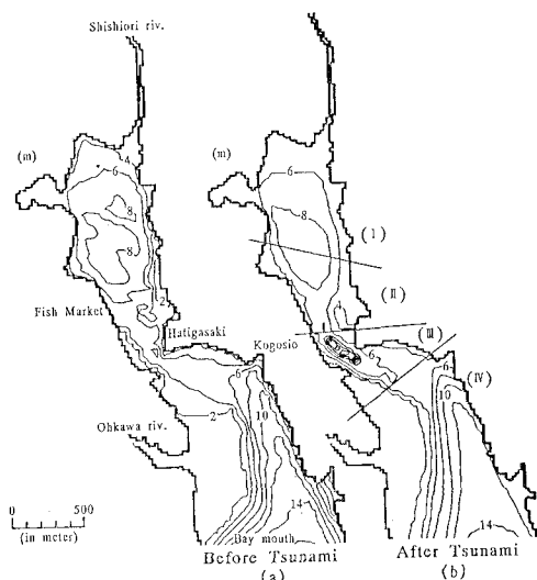
図-2 津波前と津波後の水深
