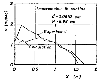
図-4 そ上速度の距離の変化
