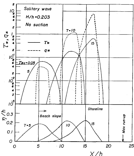
図-6 孤立波のそ上に伴う波形、無次元掃流力および無次元漂砂量の場所的変化
