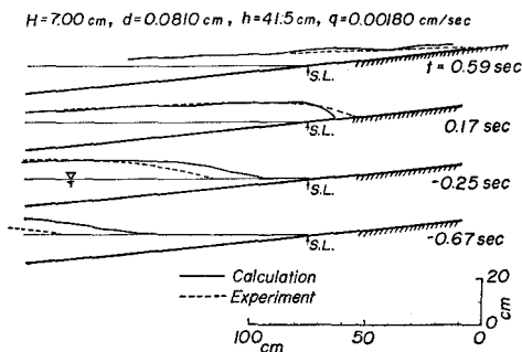
図-9 孤立波の波形変化の比較
