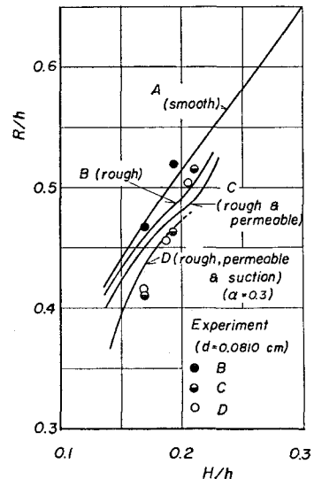
図-5 そ上高に及ぼす粗度と透水性の効果
