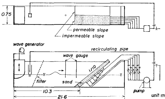
図-8 孤立波による実験装置の概略図
