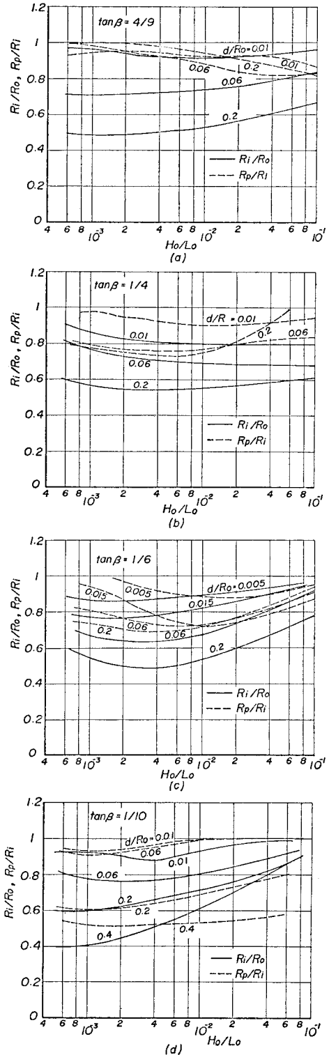
図-3 波のそ上高に及ぼす海浜の粗度と透水性の効果
