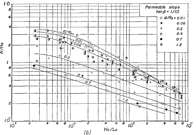
図-6 透水性海浜における波のそ上高
