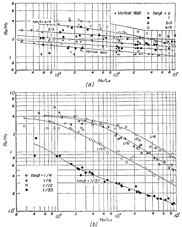
図—2 滑面の海浜における波のそ上高
