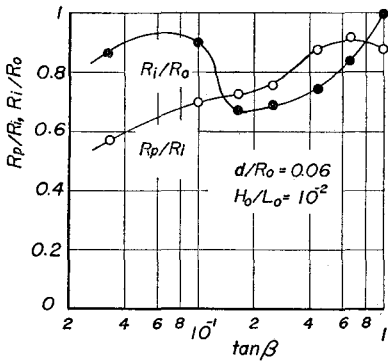
図-4 波のそ上高と海浜勾配との関係の1例
