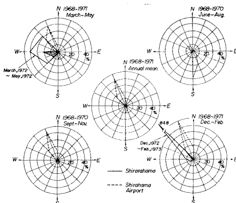
図-2 風配図
