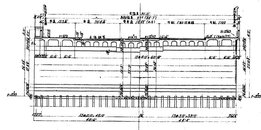
橋台部
