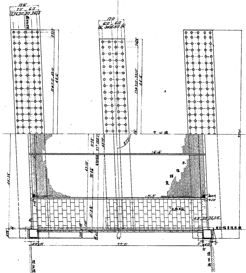
平面圖
