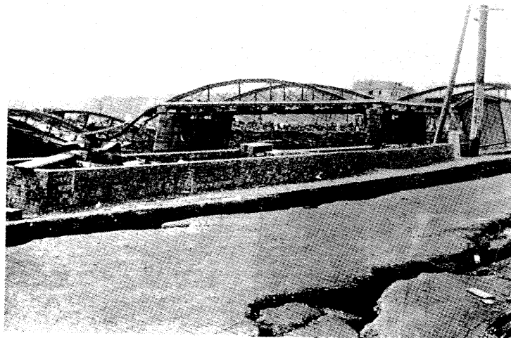
横濱市 豊國橋附近被害状況
