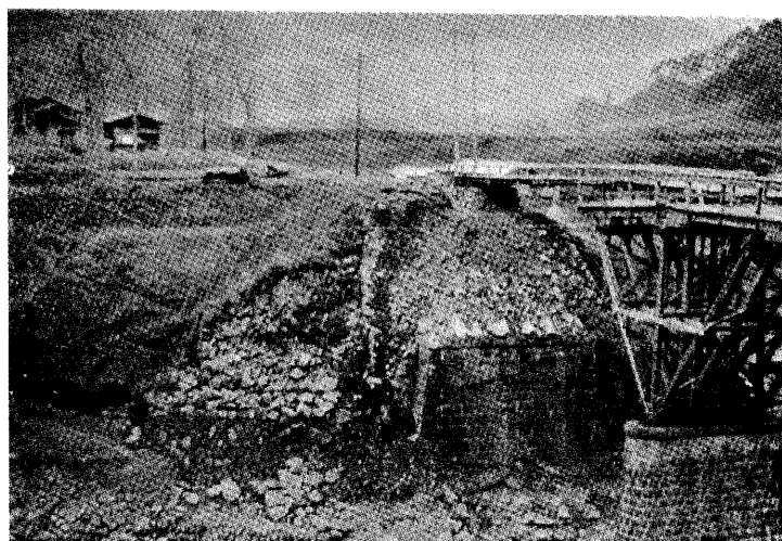
山梨縣 諸被害實況(其六)(北都留郡廣里村)
