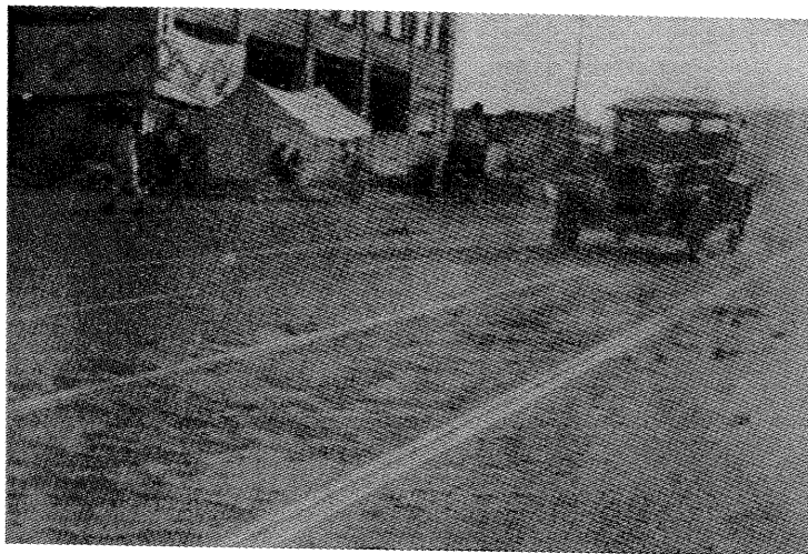
東京市 鋪木燒損狀況(銀座通り)
