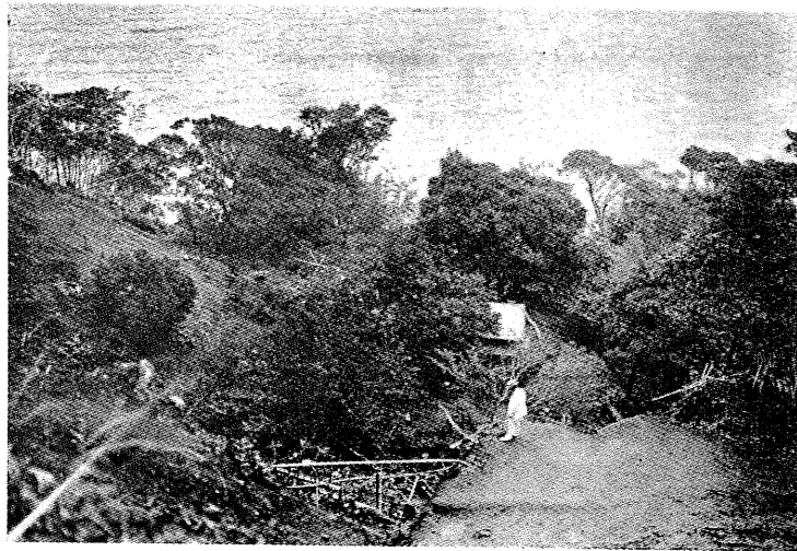
静岡県 熱海小田原線熱海町地内道路崩壊箇所(人の直立せるが道路面にしてその先に見ゆる家は元道路面の高にありしが宅地共約 80 尺の地滑を生じたるも家はその儘存せり。)
