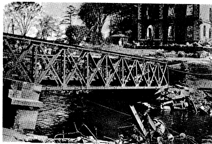
横濱市 谷戸橋被害状況
