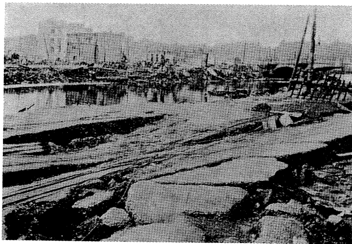
横浜市 港町河岸道路被害狀況
