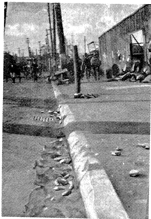
東京市 道路側溝焼損状況
