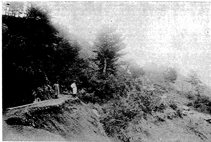
静岡県 熱海小田原線熱海町地内道路崩壊箇所(2人の直立せる箇所は舊道路面にして道路及び電柱は山と共に約 20 尺下に滑り落ち地割を生ず。)
