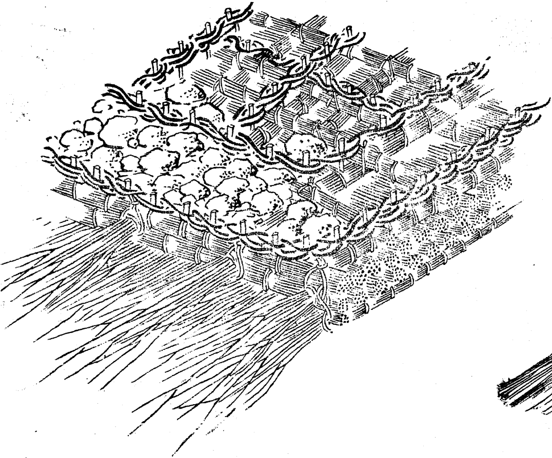
扇狀工ニ石ヲ詰タル 部分ヲ掲ケル圖
