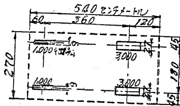
第二種 (八トン)
