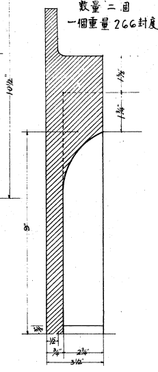
永代橋高欄及排氣傘覆詳細
