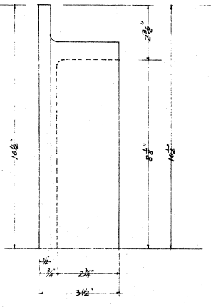
排氣傘鑄鐵架覆詳細
