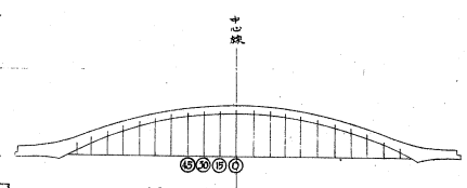
永代橋 中央徑間 (突折繫拱) 吊棧
