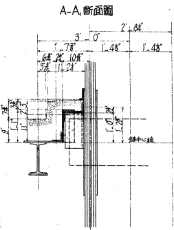
A-A断面圖
