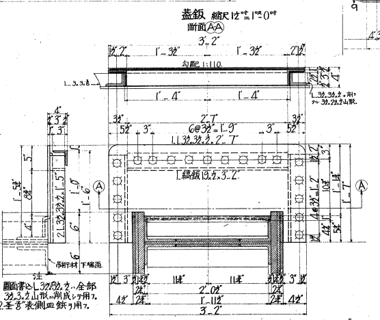
永代橋 中央徑間(突桁繫拱) 繫材取附詳細圖
