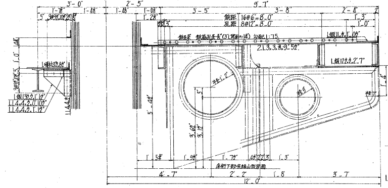
B-B断面圖
