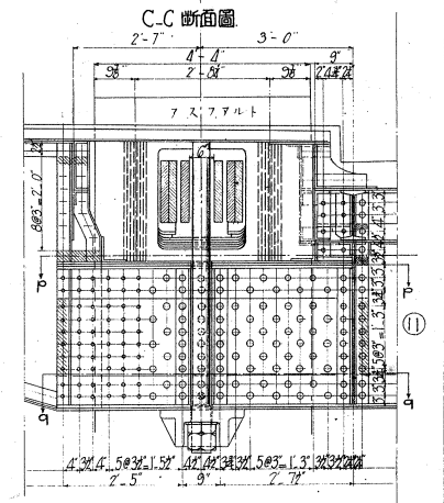
永代橋 中央徑間(突桁繫拱) 繫材取附詳細圖
