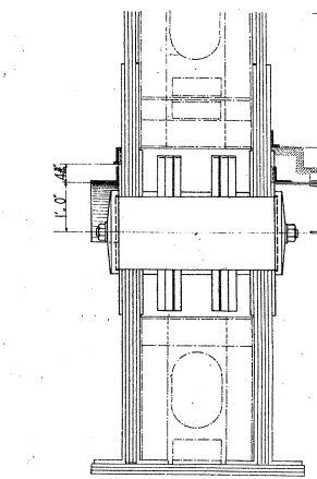
A-A断面圖
