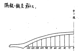
永代橋 中央徑間(突桁繫拱) 支間 { 繫拱 1.330° (突拱 2.47°) 断面詳細圖
