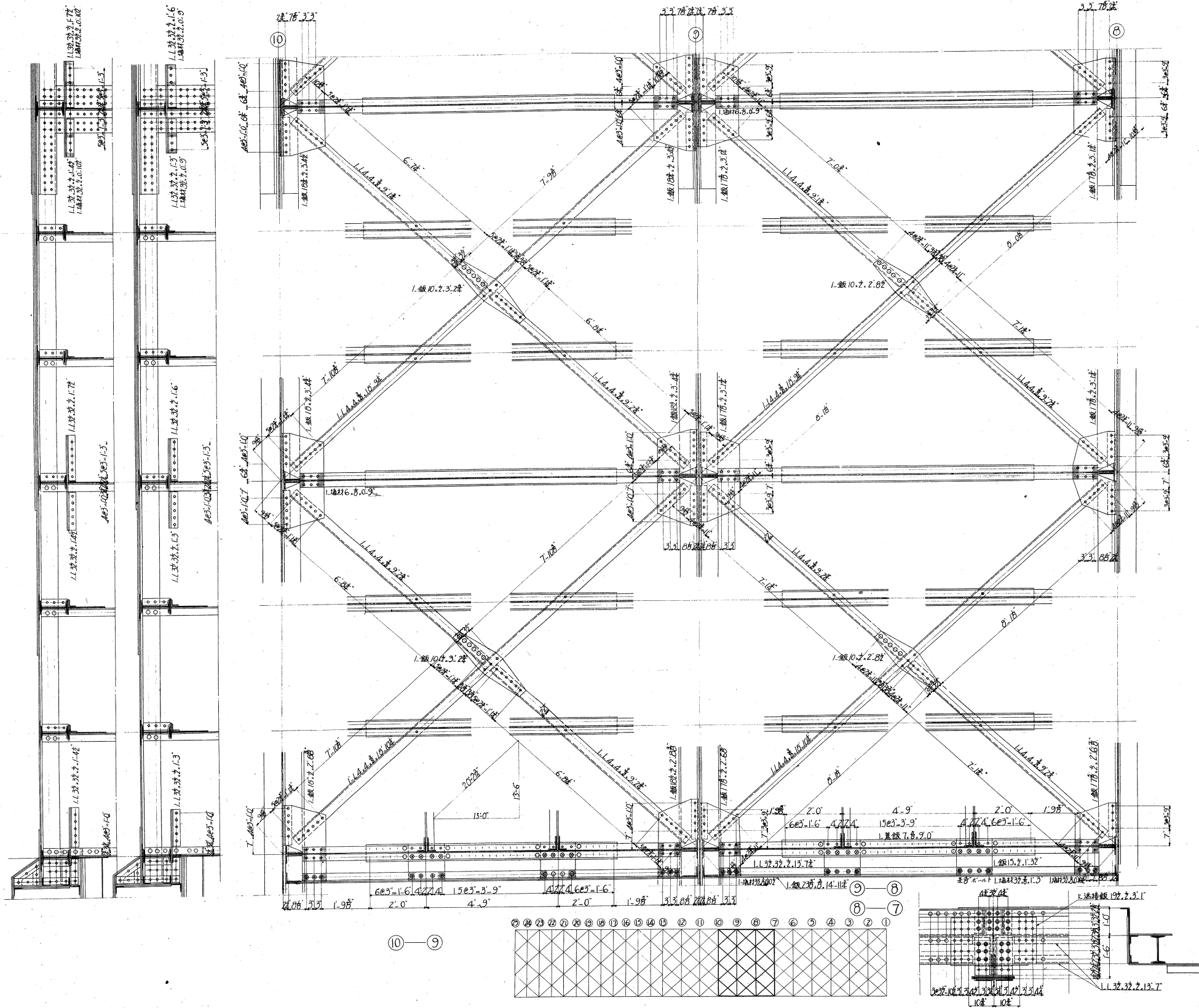
永代橋 下構
