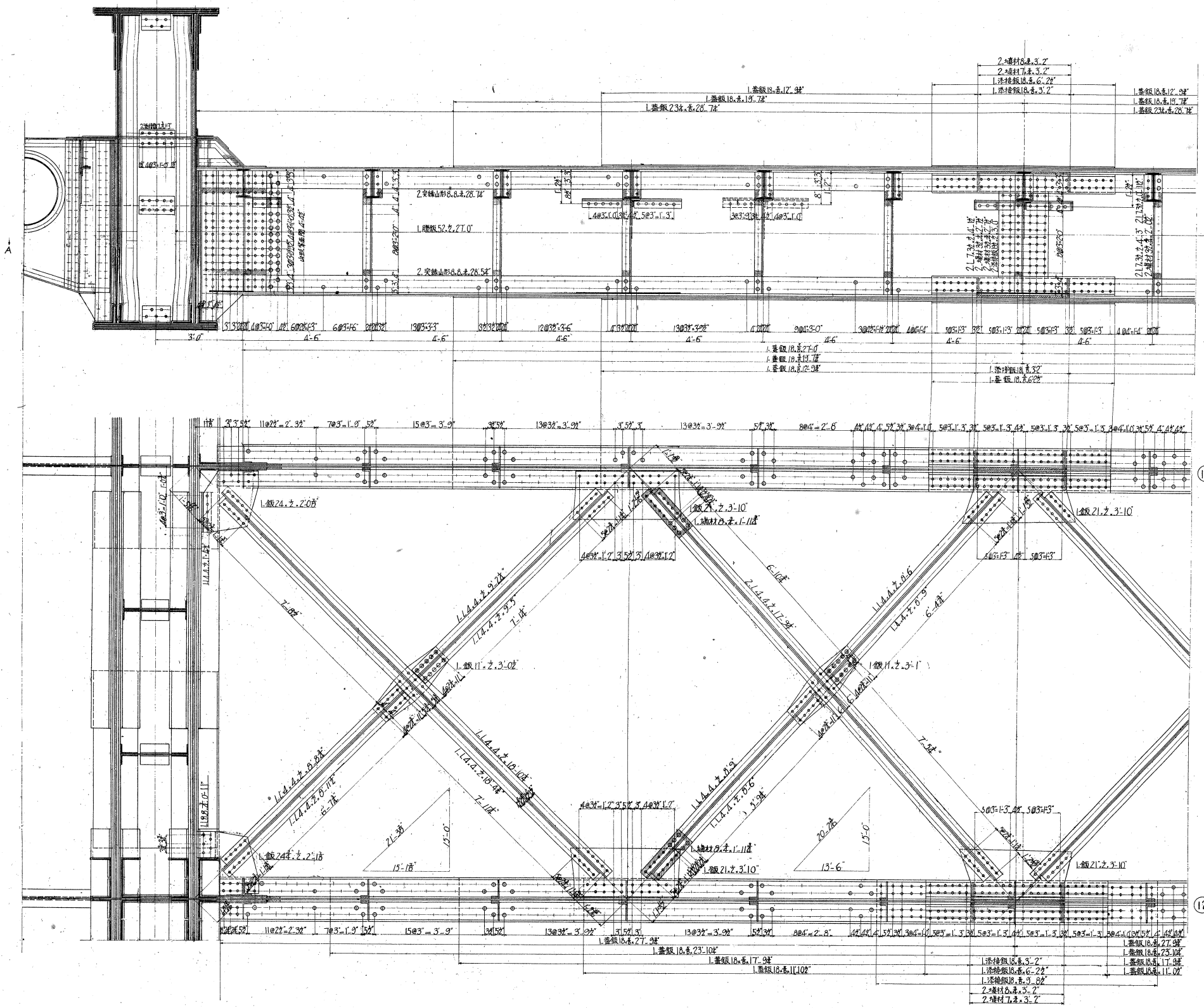
永代橋 下構
