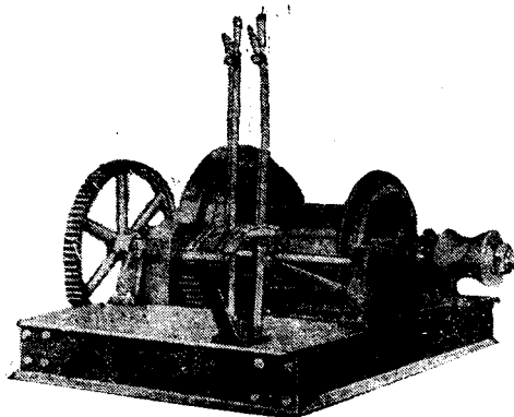
田中式捲揚機
