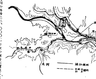
渡川改修工事平面圖 建設技官 三好宗逸
