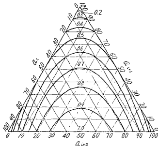
図-14 粒度の標準偏差の範囲 (4成分の場合)
