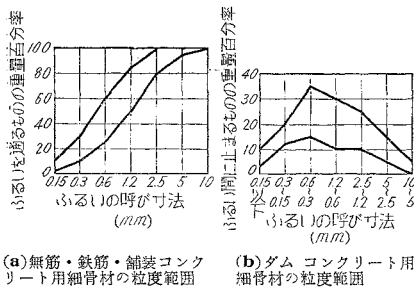
図-1 骨材の粒度を表わす2つの方法
