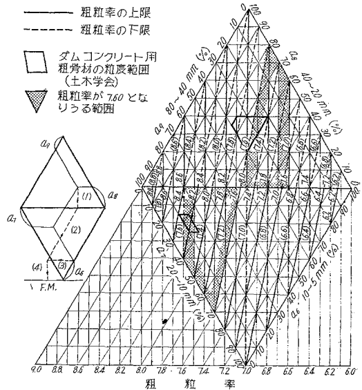
図-5 粗粒率の求めかたと粗粒率の範囲 (4成分の場合)
