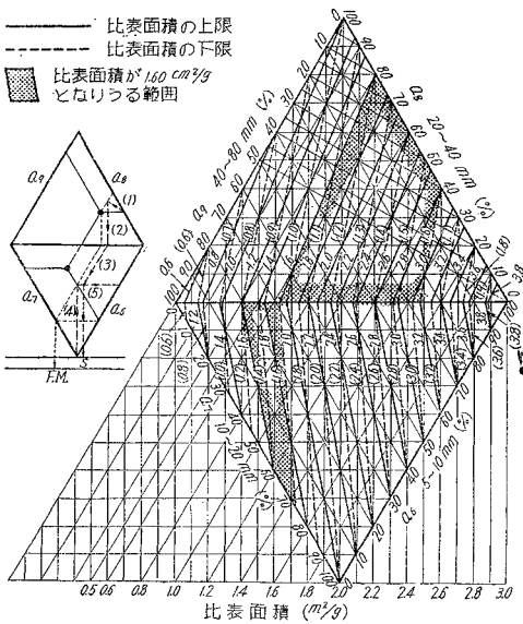
図-10 比表面積の求めかたと比表面積の範囲 (4成分の場合)
