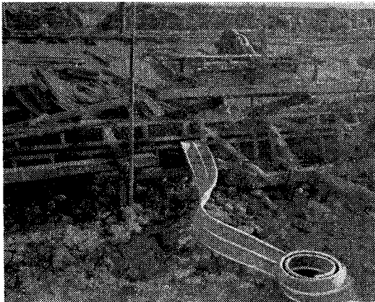
建設省伊勢湾防潮堤工事
