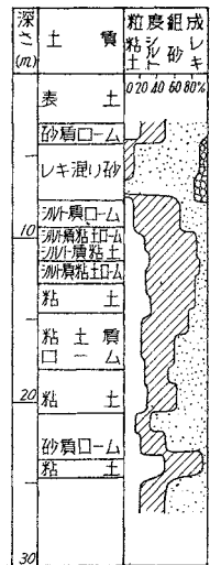
図-3 土質柱状図 (No. 30 地点)
