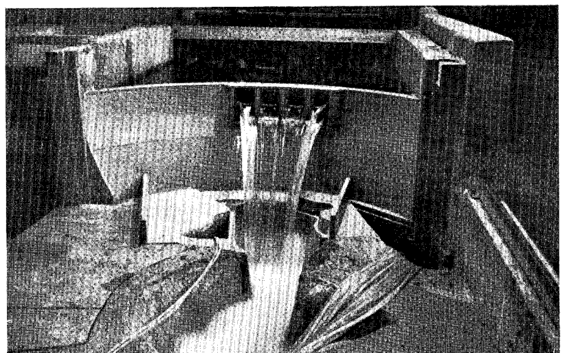
センター オーバー フロー水理実験
