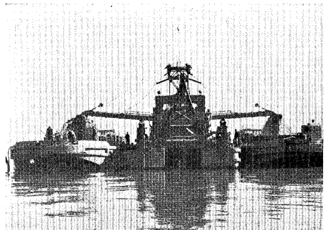
ディーゼル カッターレス しゅんせつ船“双竜”
