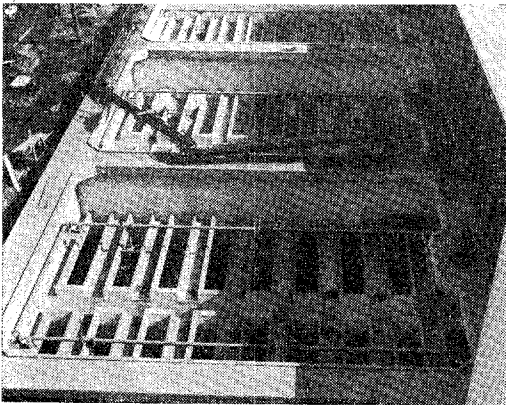
写真-7 急速ろ過池
