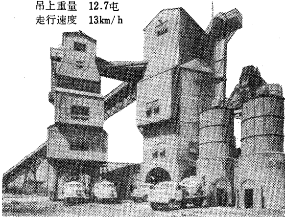
生コン用バッチャー プラント 56S ミキサー 2基
