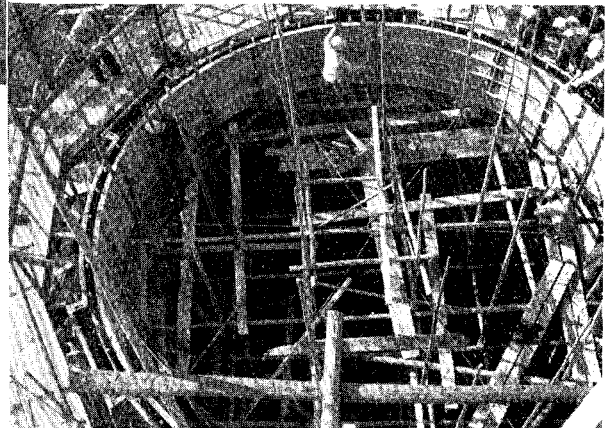
型 ワ ク 組 立 作 業
