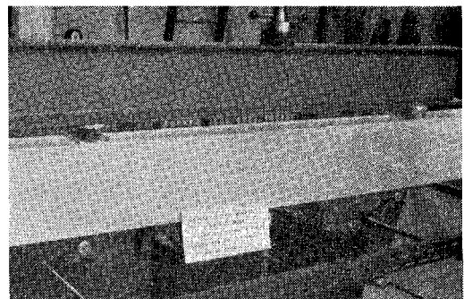
写真-3 ロンドン市外 Building Research Station コンクリート 疲労試験
