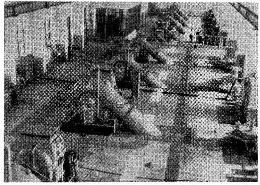
写真-6 混和池急速攪拌機および緩速攪拌機
