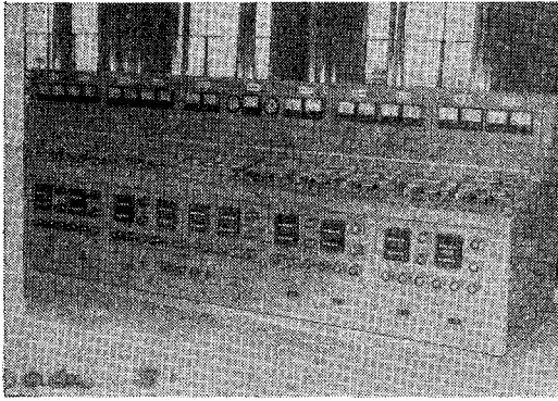
写真-4 1人制御式取送水ポンプ操作台
