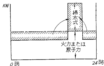
図-7 日調整揚水方式
