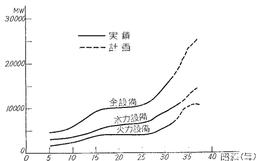
図—3 発電設備の傾向
