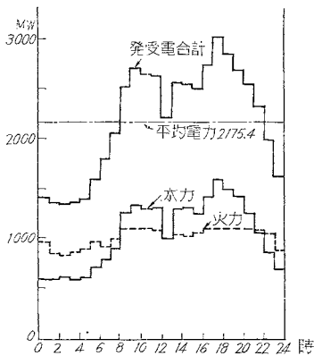
図一5 昭.32.12.18. 東京電力管内、第三水曜日負荷曲線 (負荷率 72.2%)
